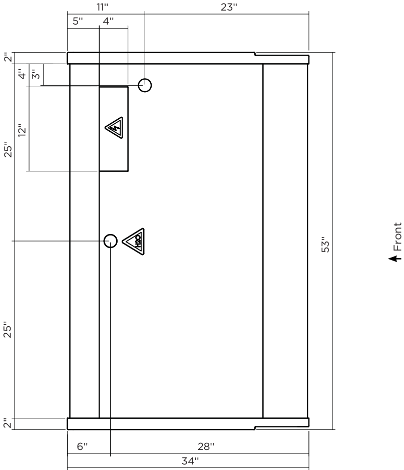
KBD-CG/FG-50-S(D)
