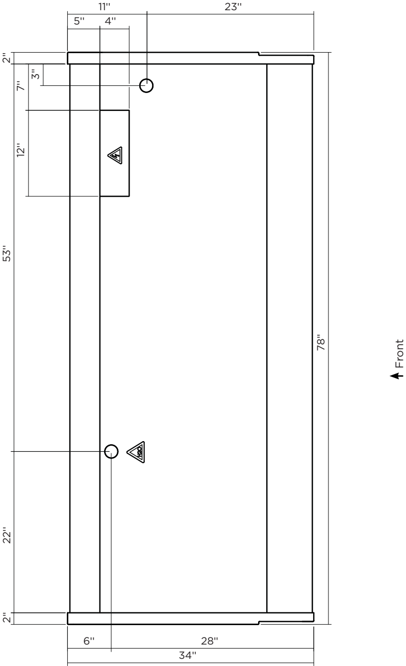
KBD-CG/FG-80-S(D)
