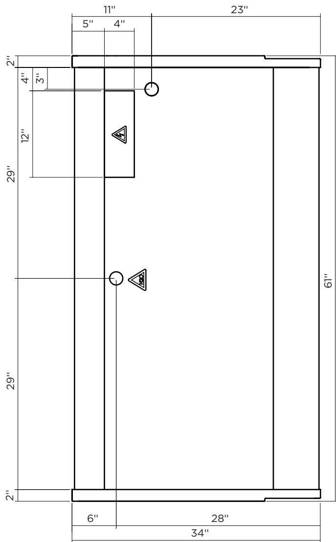
KBD-CG/FG-60-S(D)
