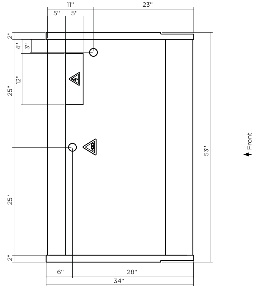
KBD-CG/FG-50-R(D)
