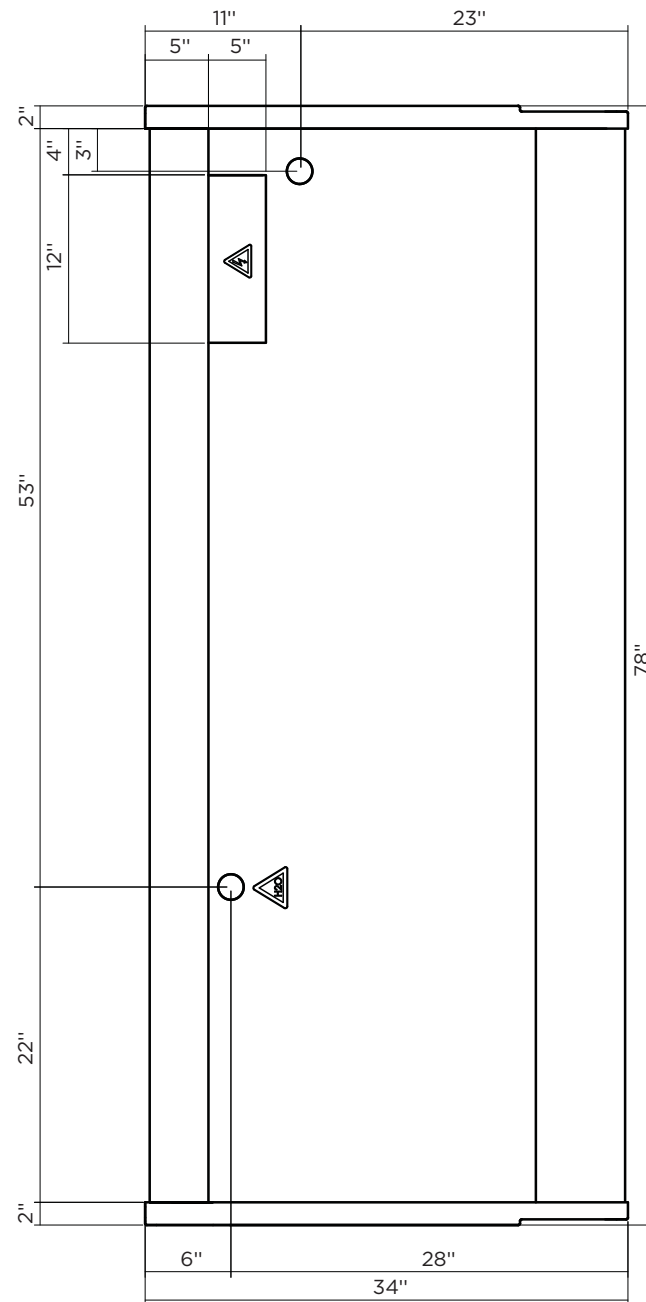
KBD-CG/FG-80-R(D)
