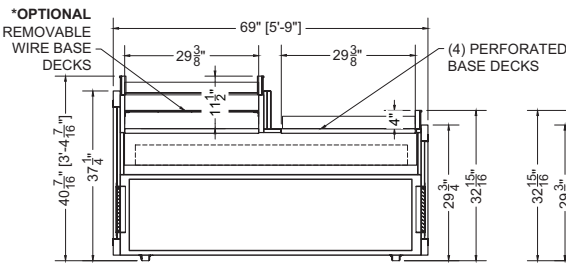
Section A:A View
