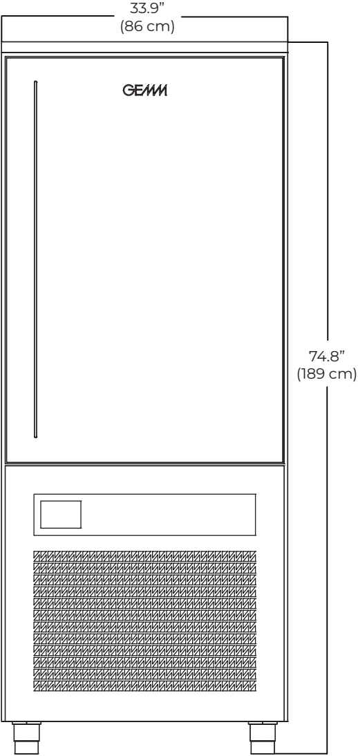
FRONTAL VIEW VUE AVANT
